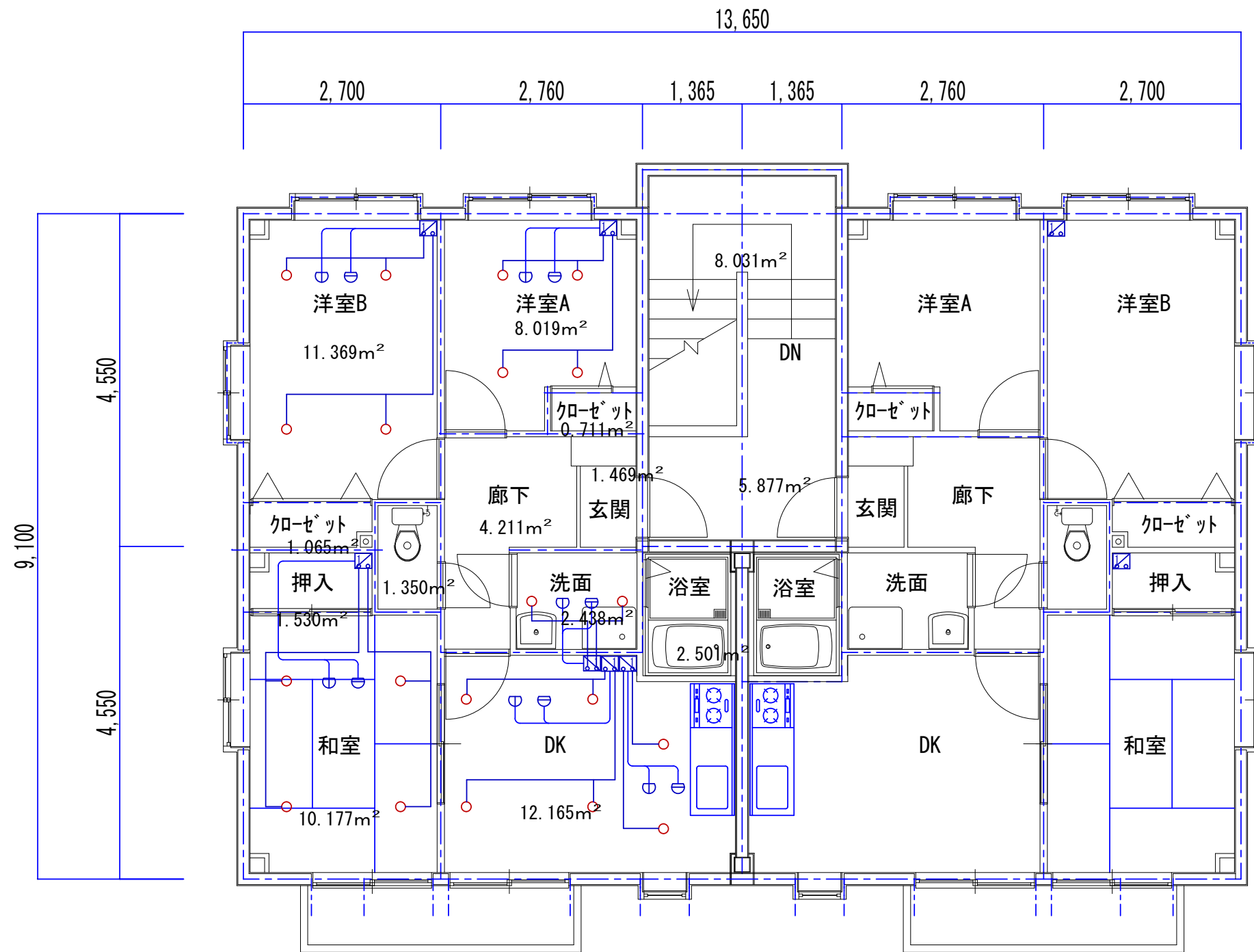
2 階平面図
