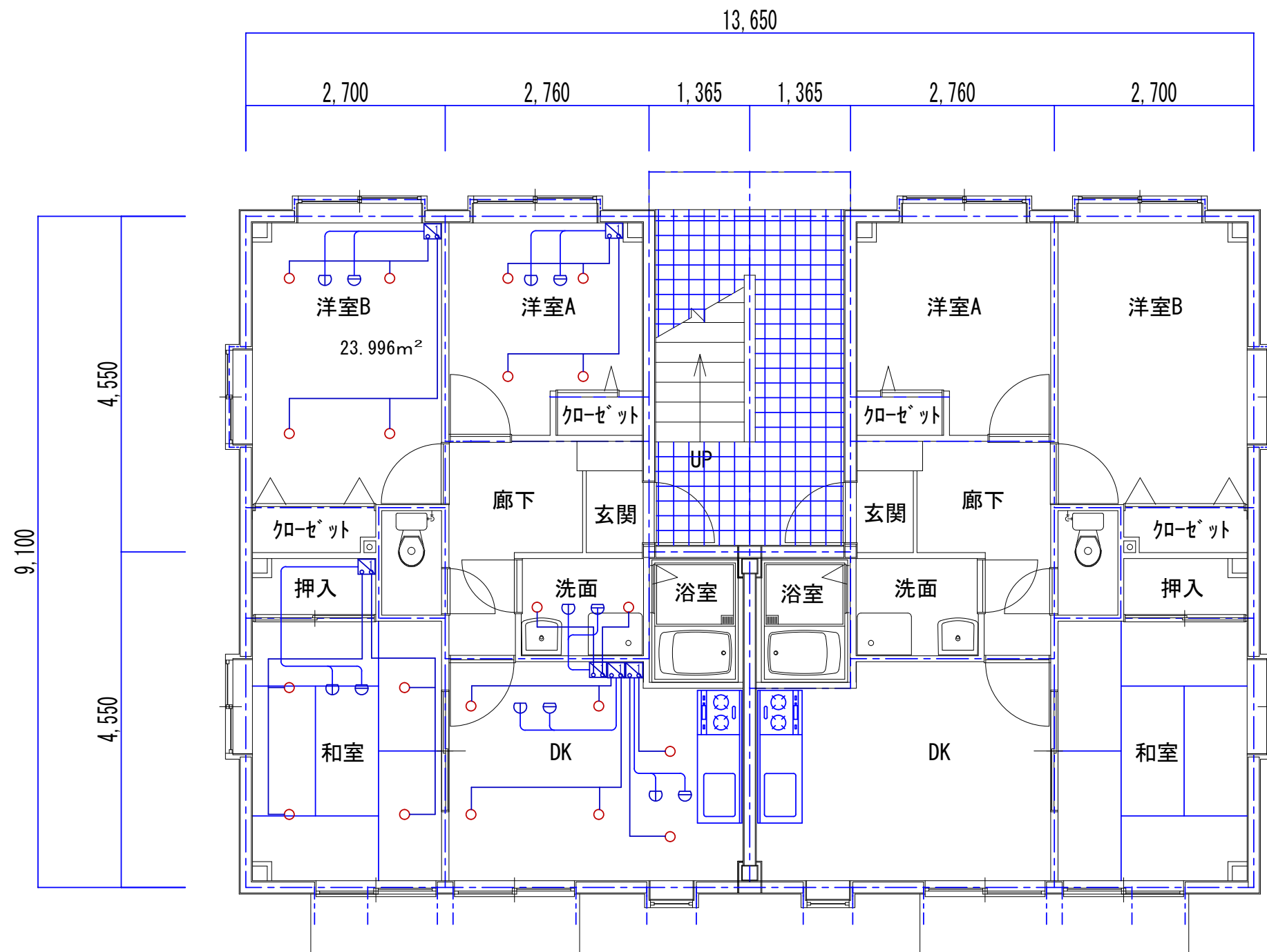
1 階平面図
