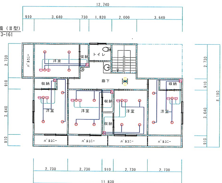
2階 平面図
