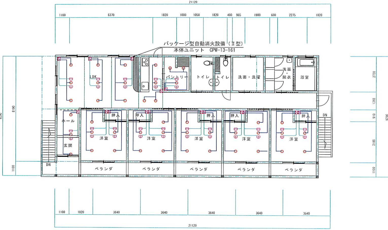
2階 平面図
