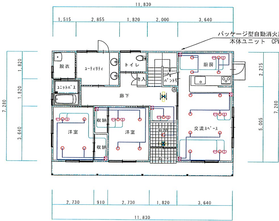
1階 平面図
