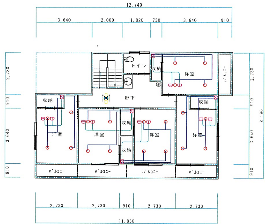
2階 平面図
