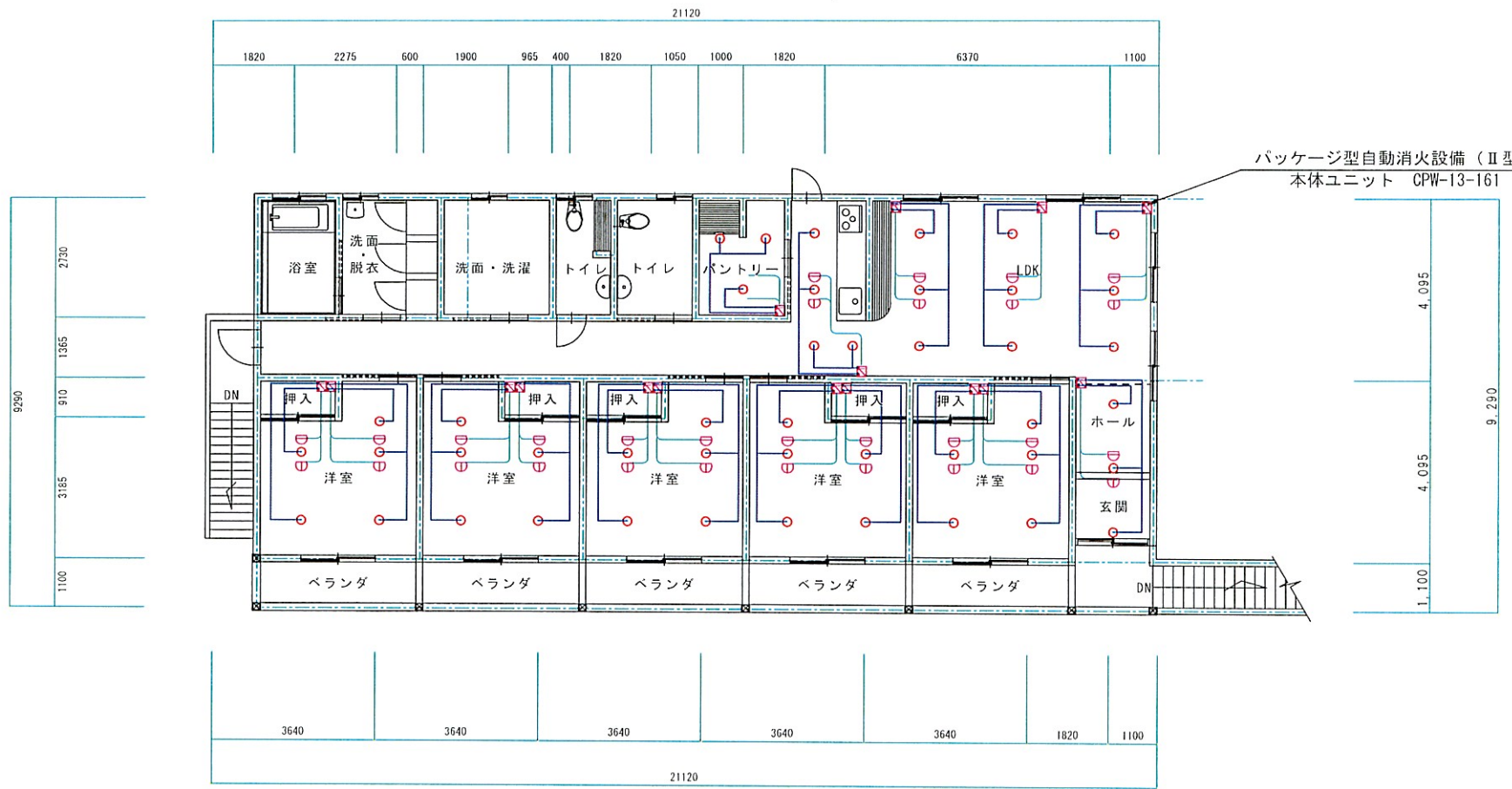
2階 平面図
