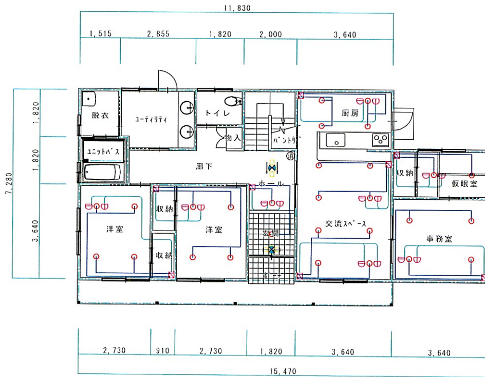
1階 平面図
