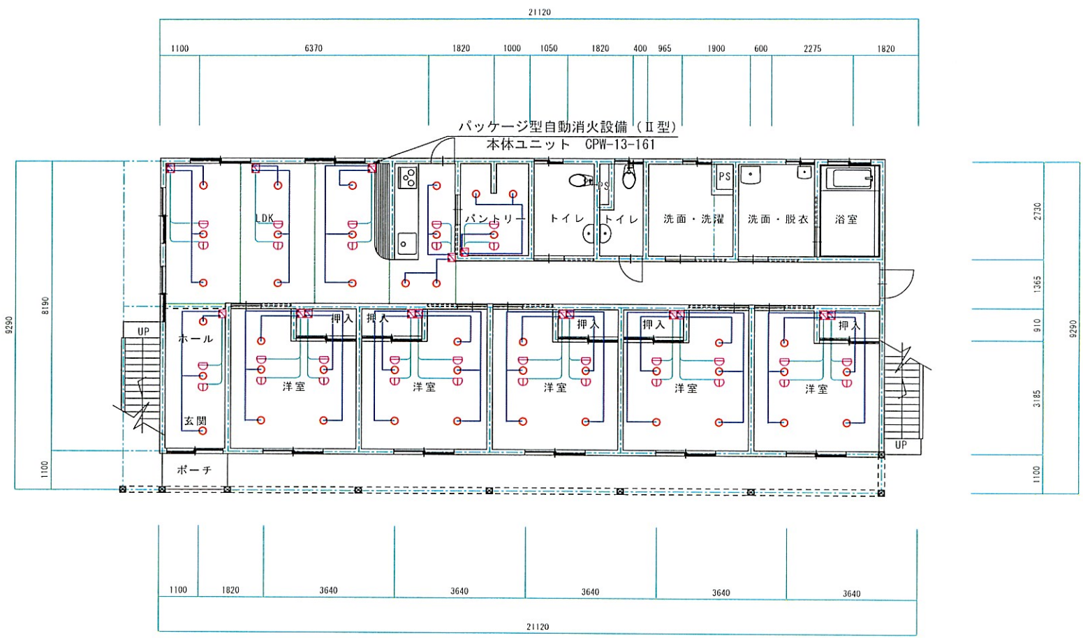
1階 平面図
