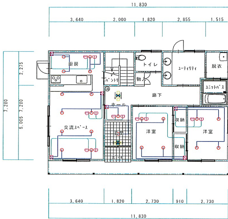
1階 平面図
