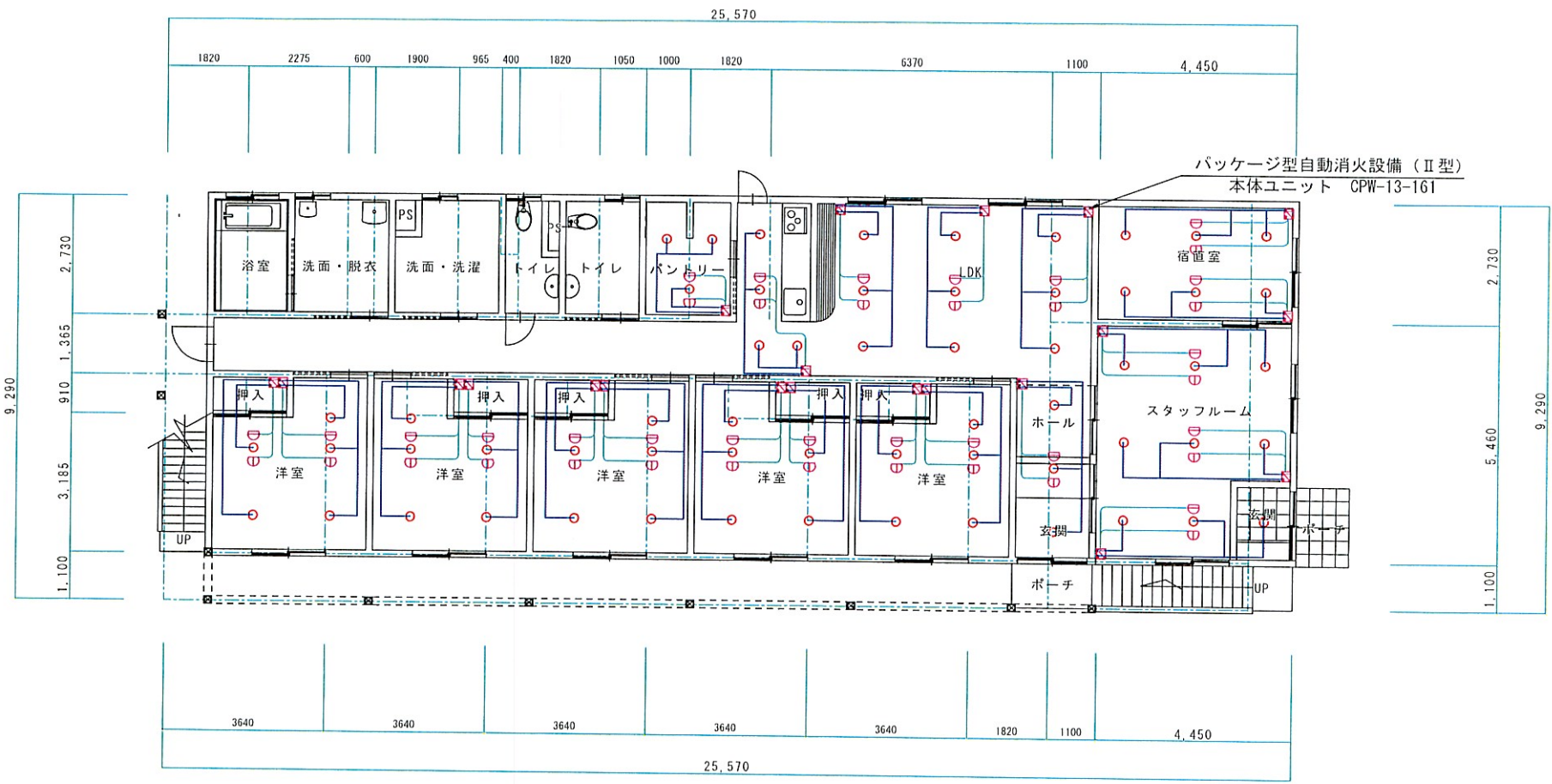
1階 平面図
