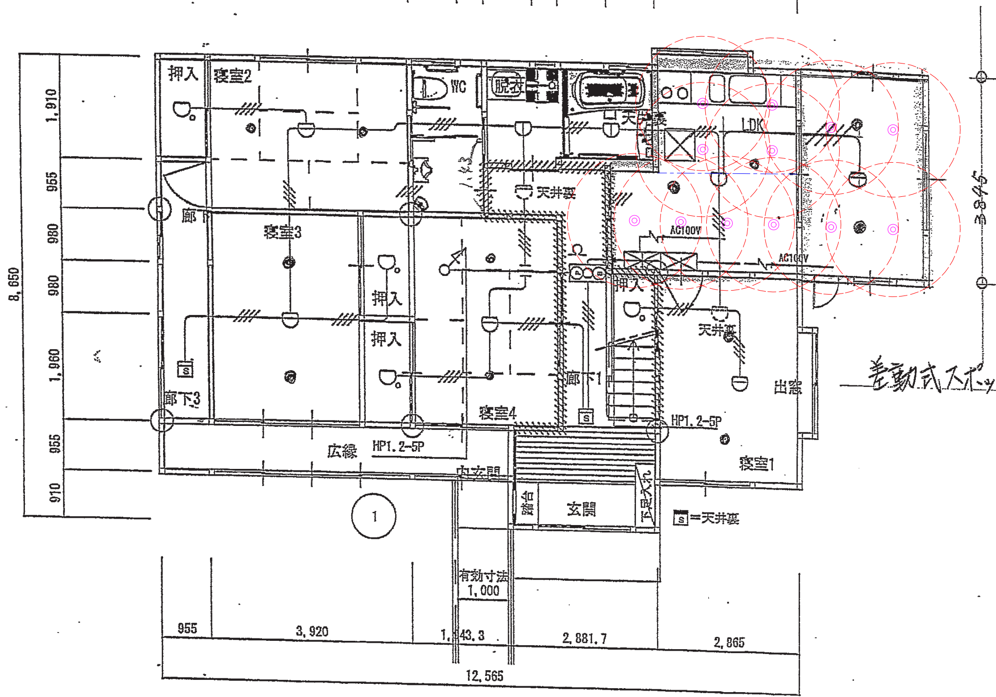
改修 1階平面図 1/100
